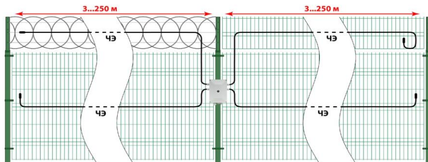
ЛИАНА
